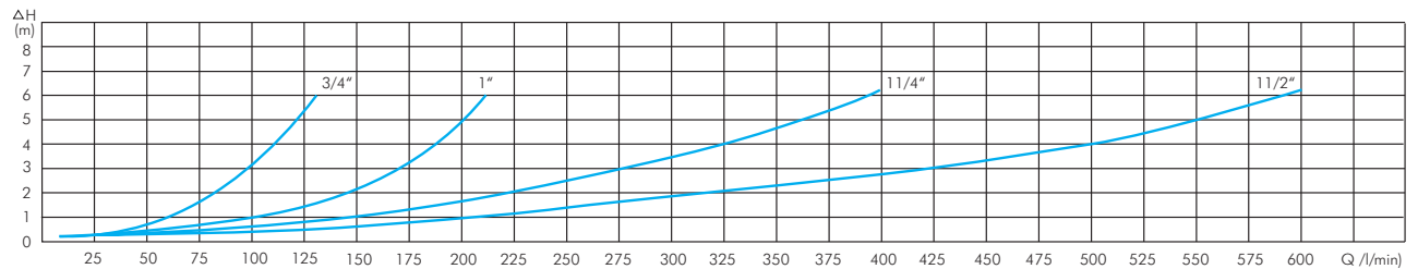
Durchfluss-Diagramm RUCK 34/10/114/112 ES / ES 4A
