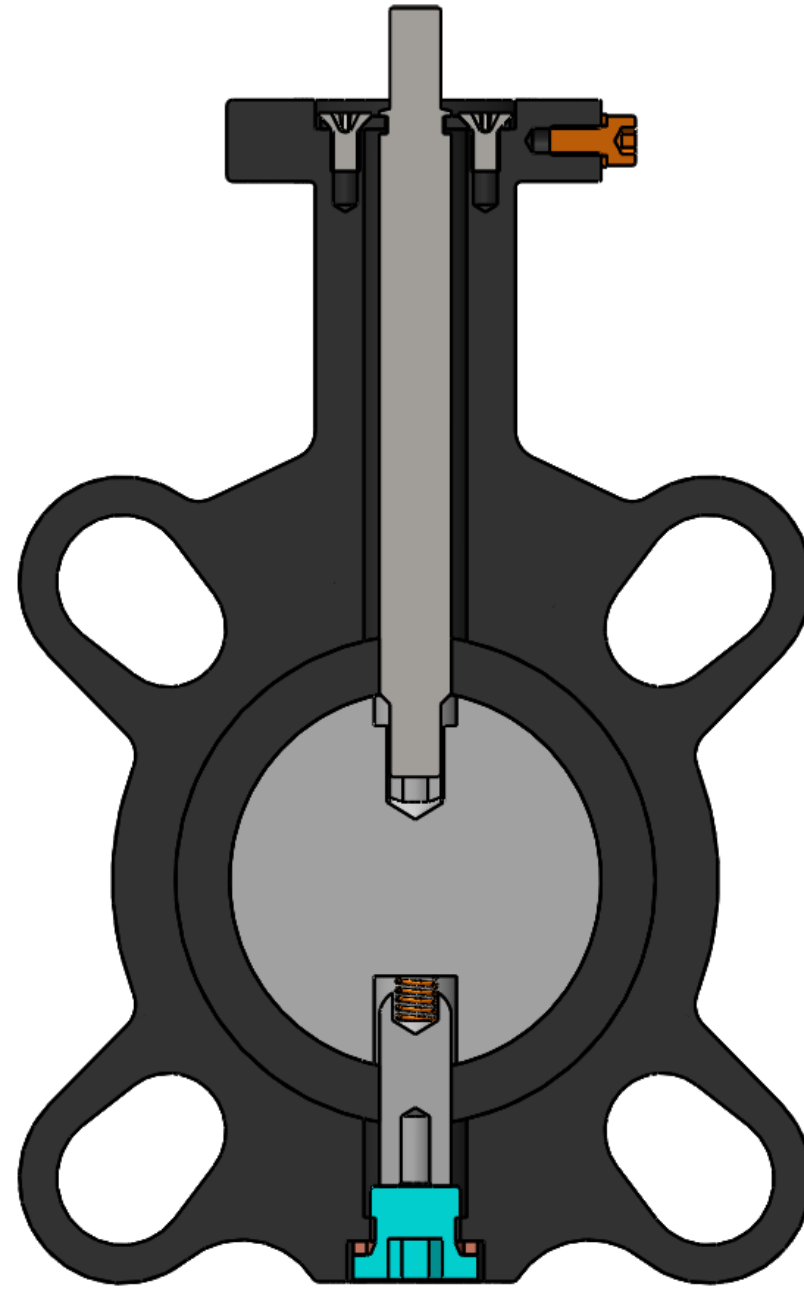
SECTION A-A SCALE 4 : 5
