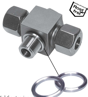
Dichtkantenring
